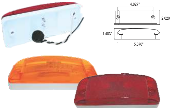
Conector. 7088
